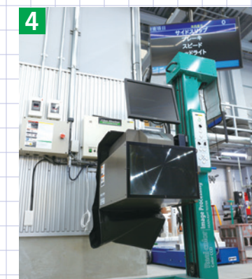
▲手動式画像処理ヘッドライトテスター“HLI-215”と視認性抜群の43インチモニター。システムは“ラインマスター”を採用
