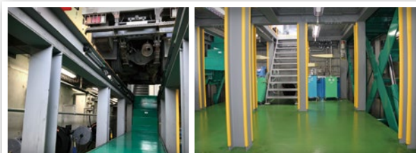
▲2基の“フロアリフト”の地下ピットを連結させて、分解作業場として使用。オイル交換やミッション分解作業もピット内で完結
