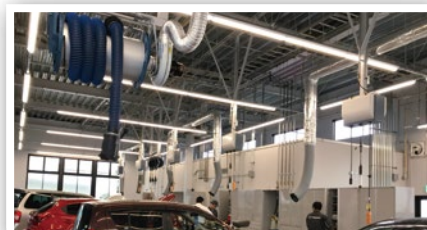
▲DPF強制燃焼時の対策として排気ダクトを設置。各ストールにはスポットクーラーも設置されメカニックの働きやすい作業環境づくりに注力
