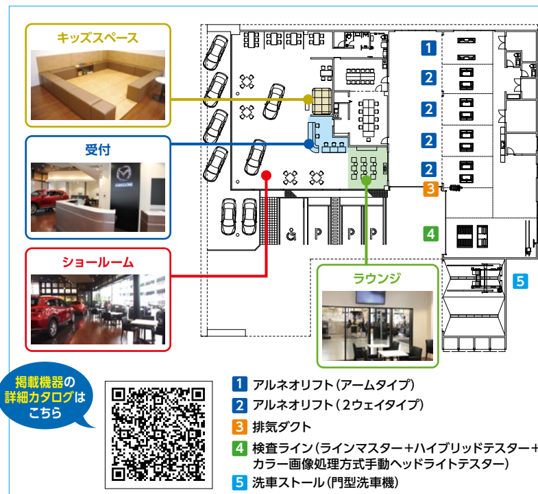
▲最新設備を導入し、ユーザーニーズに応えるため万全の態勢を整えた検査ライン。検査業務の効率化が期待される
