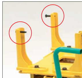
爪部はボルト固定フリータイプのため、小型～大型まで多様なミッションに対応 爪部の金属面が直接ミッションに当たらないゴムパット(オプション)を用意
