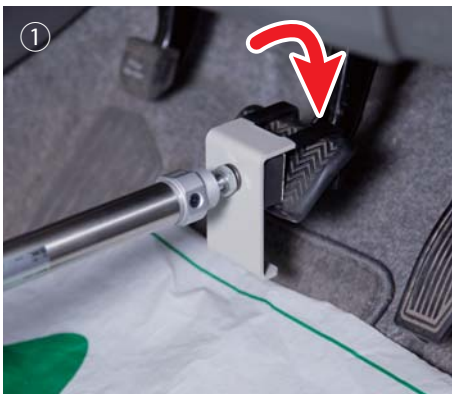
① ブレーキペダルにペダルホルダーを引っ掛けます。
