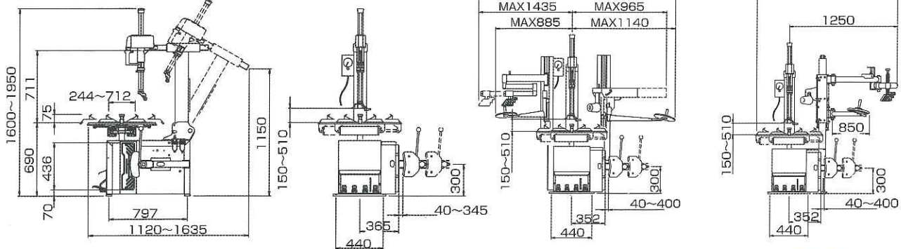
HELP&プレスアーム取付時
