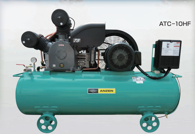
■タンクマウントタイプ ATCシリーズ
