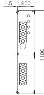
外観図は、ABS-212 ABS-210S/210/206S/206も同寸法
