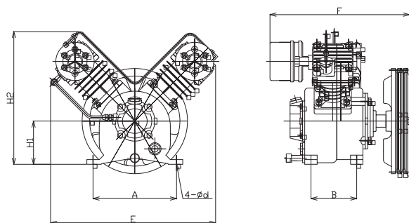
寸法図 OF-22～OW-110L
