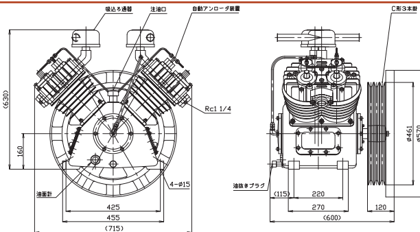
寸法図
