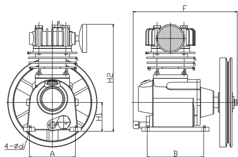
寸法図 OF-04N～OF-15
