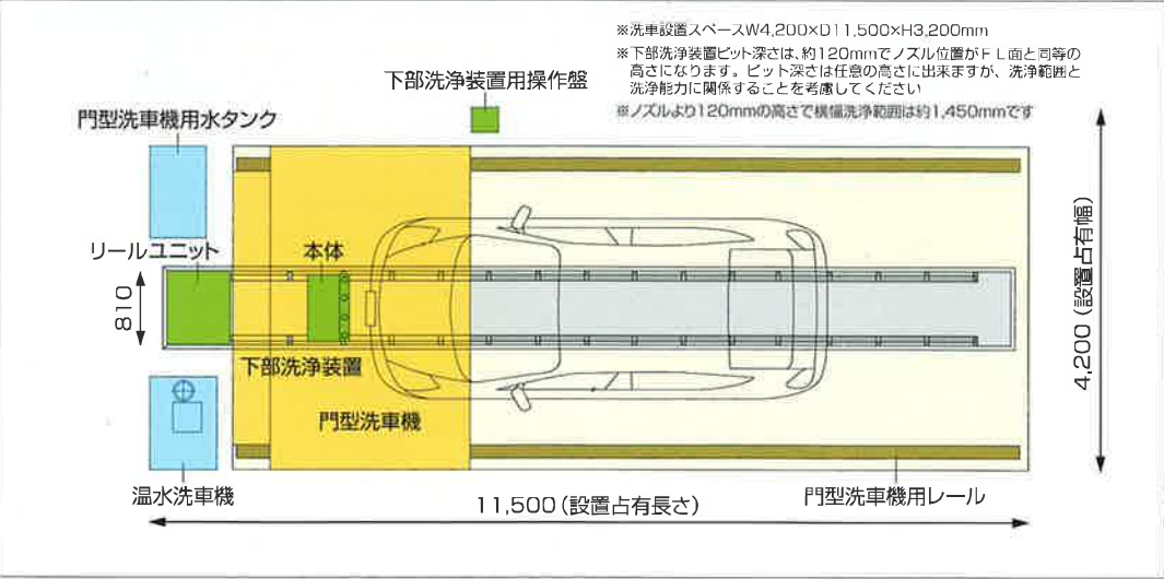
■門型洗車機&下部洗浄装置 車両自走型 参考設置図
