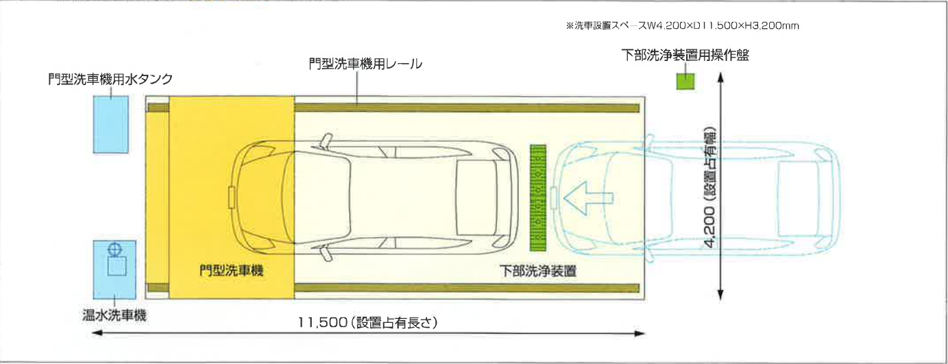
■下部洗浄装置 ハイクロールウォッシャー仕様
