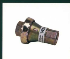
■空気圧レギュレータ ZU-074 最大圧力：1.8Mpa/18kgf/cm 2 調整範囲：0.5Mpa/5.2kgf/cm 2
