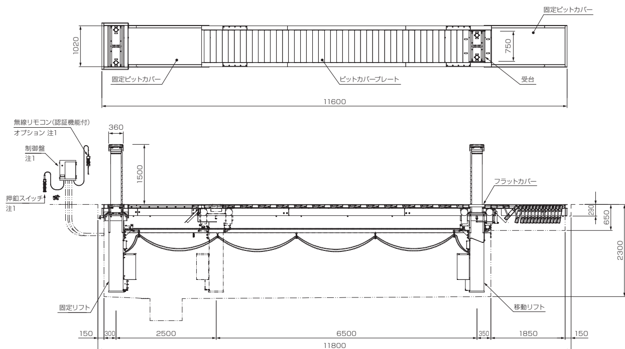
外観図はTWP30N-65 注1:無線仕様(オプション)は専用の制御盤となり、押釦スイッチは付属しません
