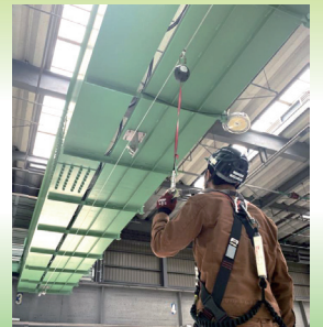
荷台からの転落を防ぐ 常設型 転落防止システム アクロバット
